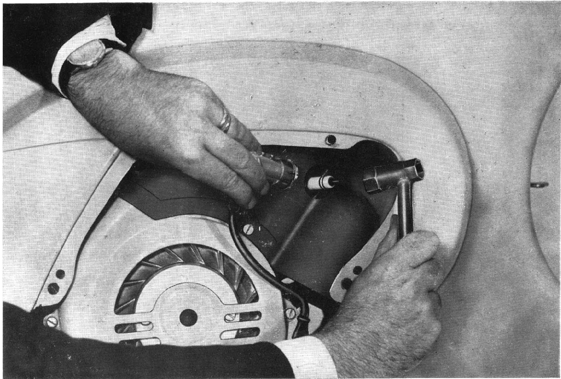
Fig. 13 - Desmontaje de la bujía
